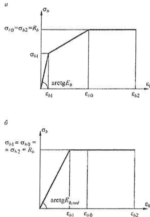
а – трехлинейная диаграмма состояния сжатого бетона; б – двухлинейная диаграмма состояния сжатого бетона Рисунок 5.1 – Диаграммы состояния сжатого бетона
